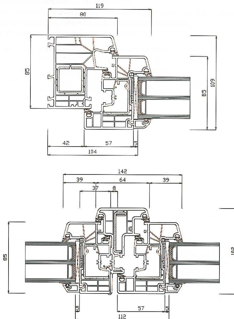
Obrázek 1 – Řez oknem
