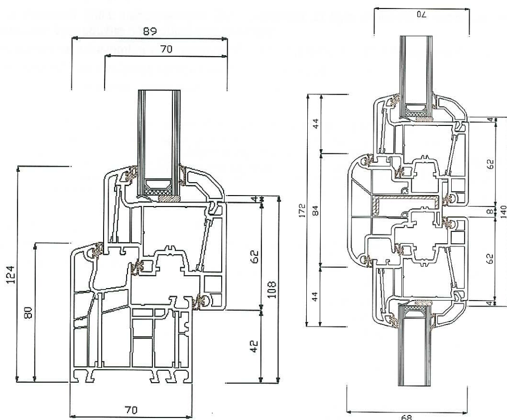
Obrázek 1 – Řez oknem
