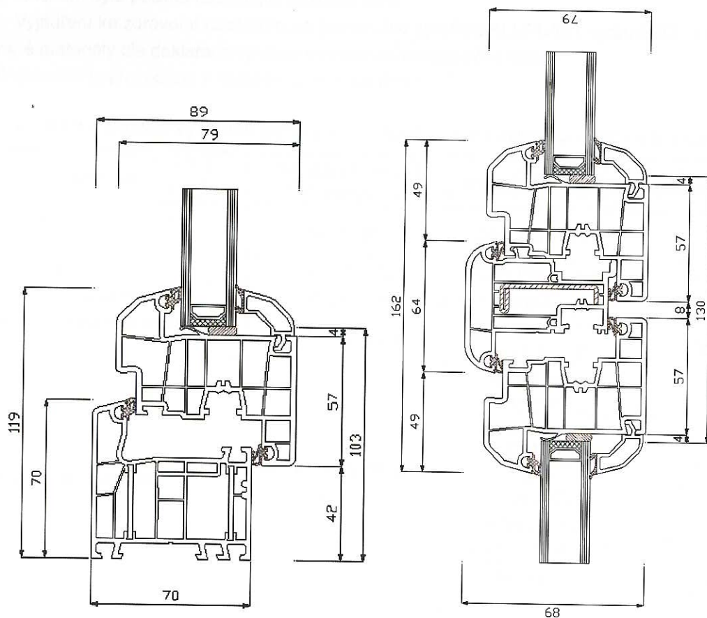
Obrázek 1 – Řez oknem
